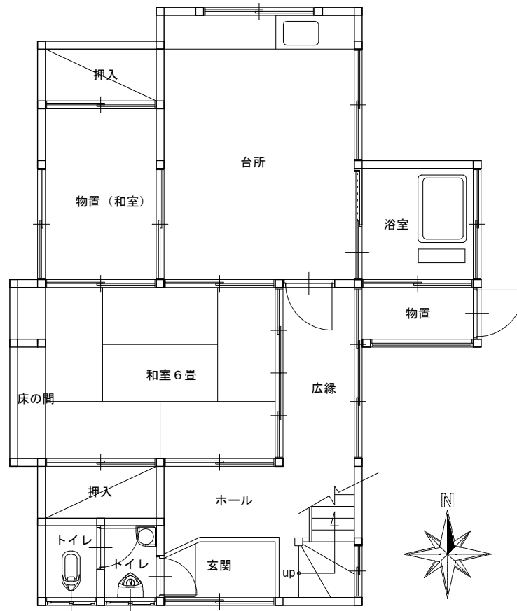
1 F 平面図
