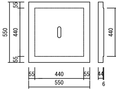
(550×550×50) <給水栓柵用蓋>
