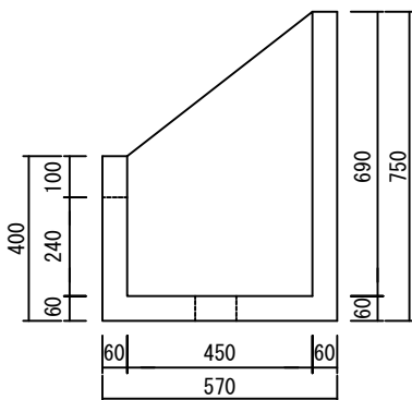
<側面図>
