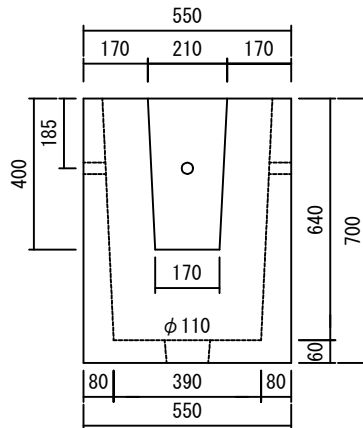
<正面図>
