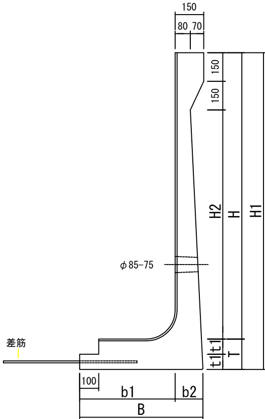
側面図
