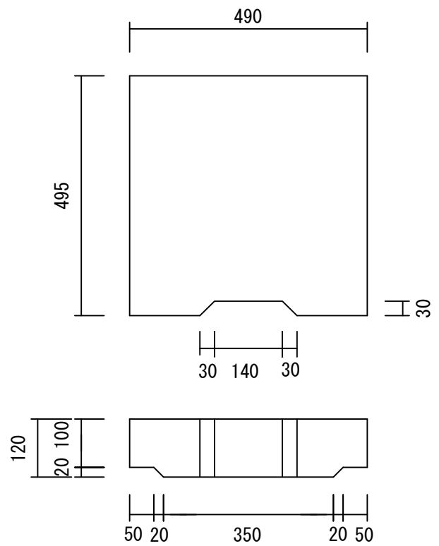
車道用 (CHL25-40) 67kg/枚
