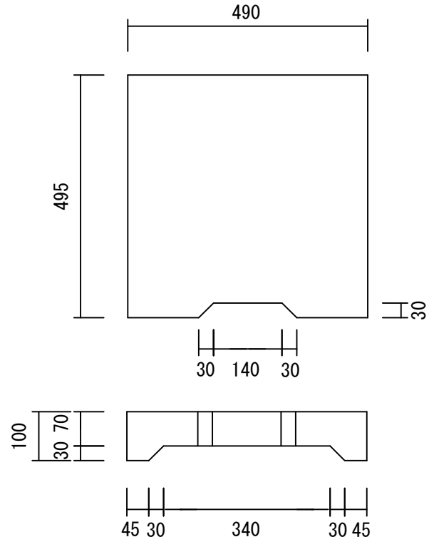
歩道用 (CHL1-40) 46kg/枚
