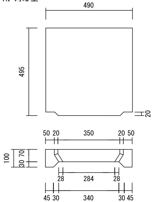
歩道用 (CHL1-40) 46kg/枚
