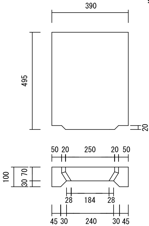
歩道用 (CHL1-30) 37kg/枚
