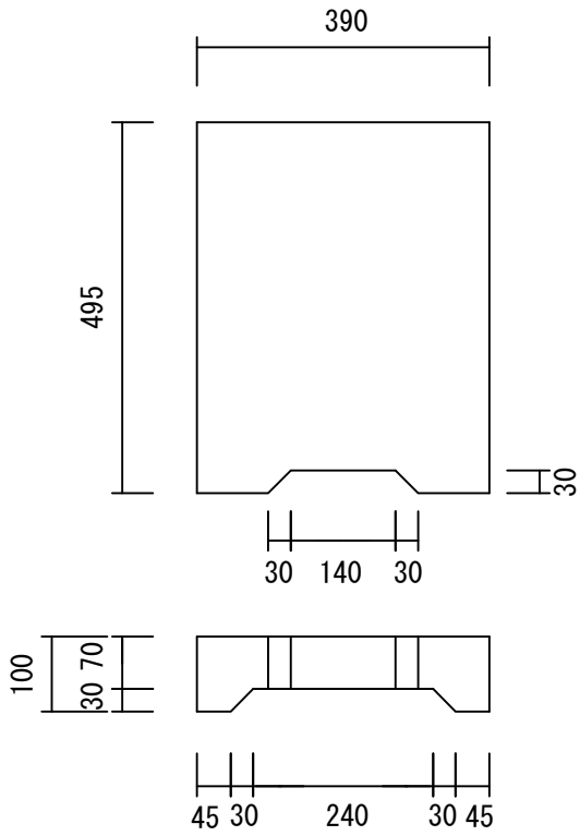
歩道用 (CHL1-30) 37kg/枚
