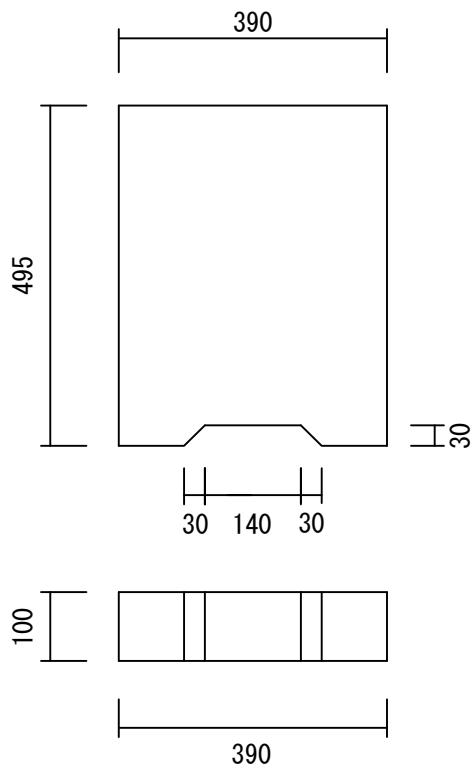
車道用 (CHL25-30) 46kg/枚
