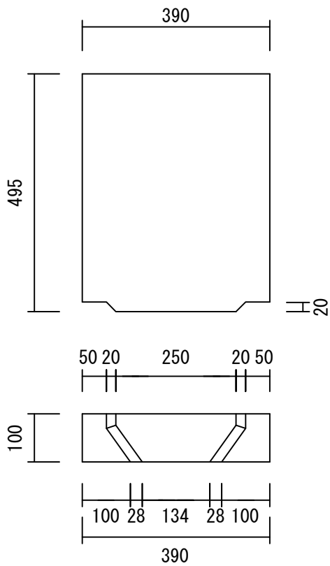
歩道用 (CHL1-30) 37kg/枚
