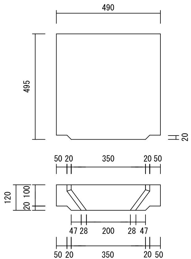
車道用 (CHL25-40) 67kg/枚
