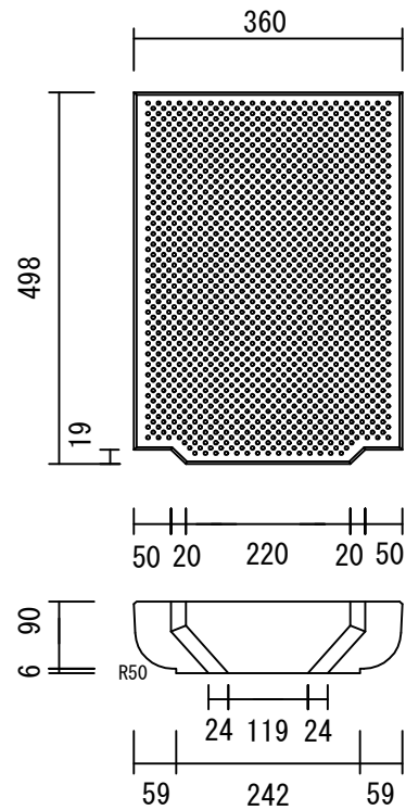
250用 ノンスリップ(ノスキッド模様) 39kg/枚
