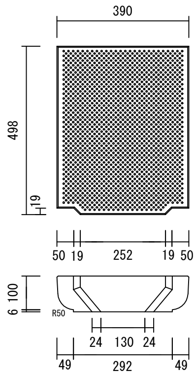
300用 ノンスリップ(ノスキッド模様) 47kg/枚
